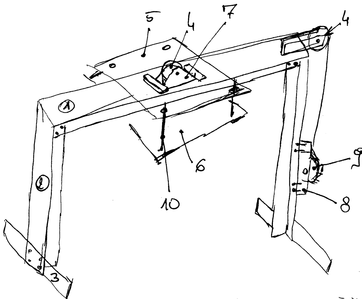
Schemat stanowiska badawczego
